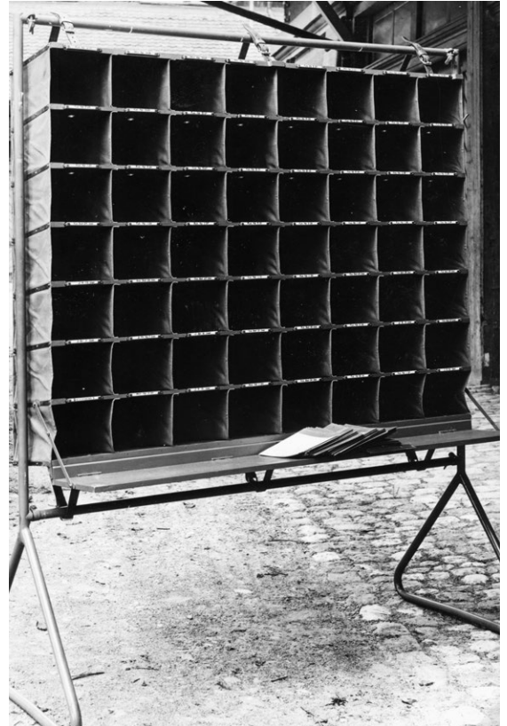
Diese mobile Ausrüstung inklusive Beleuchtung hatte in gleicher oder ähnlicher Form Bestand bis zur Auflösung der Feldpostkompanien im Jahr 2003: Brieffachgestell (Version A), 1930.
