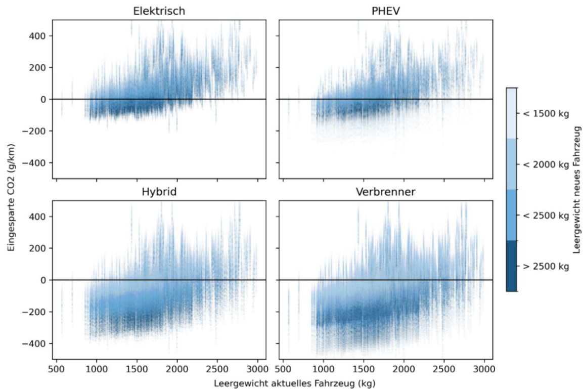
Abbildung 30: Eingesparte Treibstoffemissionen pro Kilometer für alle möglichen Fahrzeugkombinationen aus dem Verbrauchskatalog. Aktuelles Fahrzeug nur Verbrenner oder Hybrid. Neues Fahrzeug nur Modelle 2024. Antriebsart des neuen Fahrzeugs nach Quadrant. Schweizer Durchschnittstrommix. Lebensfahrlleistung 200'000 km. Graphik INFRAS.
