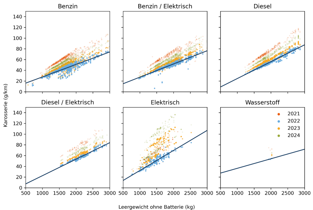
Abbildung 22: Regressionsanalyse der Karosserieherstellungsemissionen. Daten aus dem Verbrauchskatalog. Regressionsbasis: Herstellungsjahr 2022. Graphik INFRAS.
