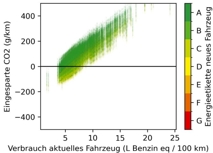
Abbildung 32: Gesparte Treibstoffemissionen pro Kilometer für alle möglichen Fahrzeugkombinationen aus dem Verbrauchskatalog. Aktuelles Fahrzeug nur Verbrenner oder Hybrid. Neues Fahrzeug nur 2024 Elektrofahrzeuge. Schweizer Durchschnittsstrommix für Elektrofahrzeuge. Lebensfahrleistung 200'000 km. Graphik INFRAS.
