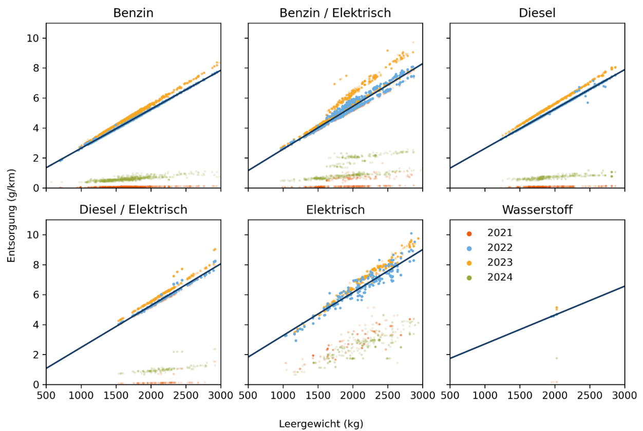
Abbildung 24: Regressionsanalyse der Entsorgungsemissionen. Daten aus dem Verbrauchskatalog. Regressionsbasis: Herstellungsjahr 2022. Graphik INFRAS.
