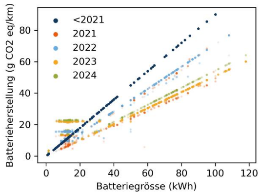
Abbildung 21: Batterieherstellungsemissionen. Daten aus dem Verbrauchskatalog. Basis für Daten vor 2021: Eigene Annahme. Graphik INFRAS.
