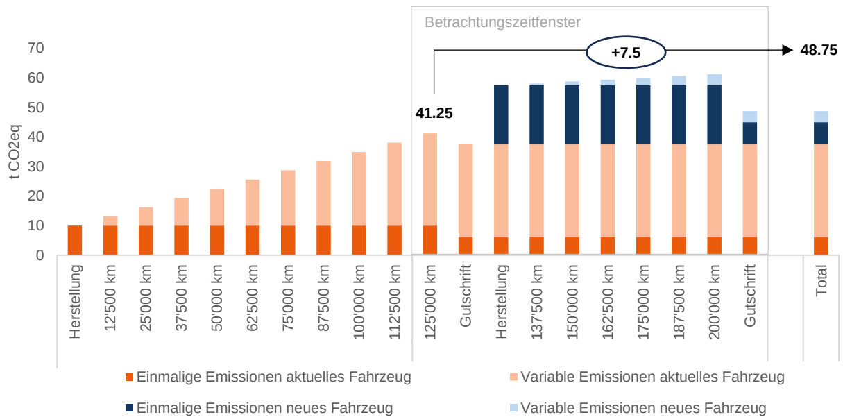
Abbildung 6: Treibhausgasemissionen Option C: Fahrzeug wird verkauft und durch ein Elektroauto ersetzt. Graphik INFRAS.
