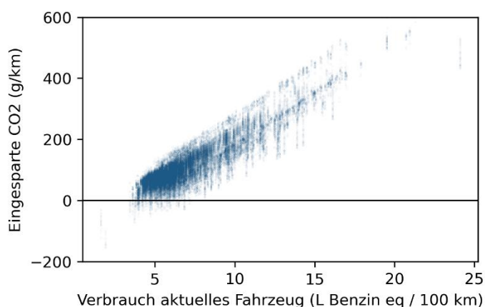
Abbildung 12: Eingesparte Treibstoffemissionen pro Kilometer für Fahrzeugkombinationen in der gleichen Fahrzeugklasse aus dem Verbrauchskatalog. Aktuelles Fahrzeug nur Verbrenner oder Hybrid mit Herstellungsjahr vor 2023. Neues Fahrzeug: Occasions-Elektroauto mit 125'000 km vor dem Kauf und Herstellungsjahr vor 2023. Schweizer Durchschnittsstrommix. Lebensfahrleistung 200'000 km. Graphik INFRAS.
