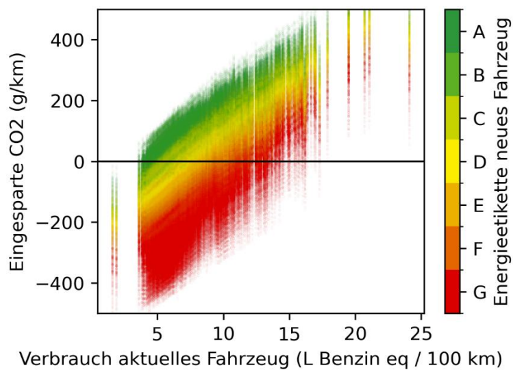
Abbildung 31: Gesparte Treibstoffemissionen pro Kilometer für alle möglichen Fahrzeugkombinationen aus dem Verbrauchskatalog. Aktuelles Fahrzeug nur Verbrenner oder Hybrid. Neues Fahrzeug nur 2024 Modelle. Schweizer Durchschnittsstrommix für Elektrofahrzeuge. Lebensfahrleistung 200'000 km. Graphik INFRAS.
