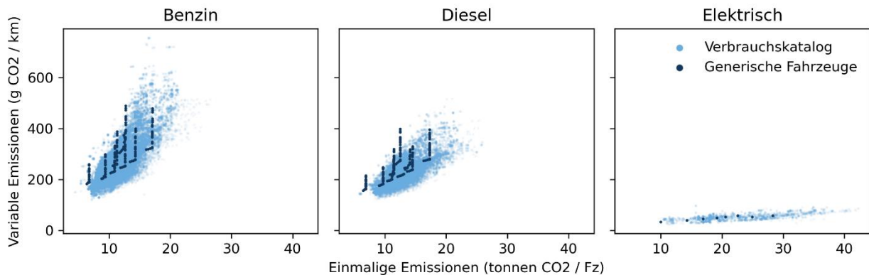
Abbildung 2: LCA-Daten für alle Benzin-, Diesel- und Elektrofahrzeuge: Verbrauchskatalog (hellblau) und generische Fahrzeuge (dunkelblau). Elektrofahrzeuge mit dem Schweizer Durchschnittstrommix geladen. Graphik INFRAS.
