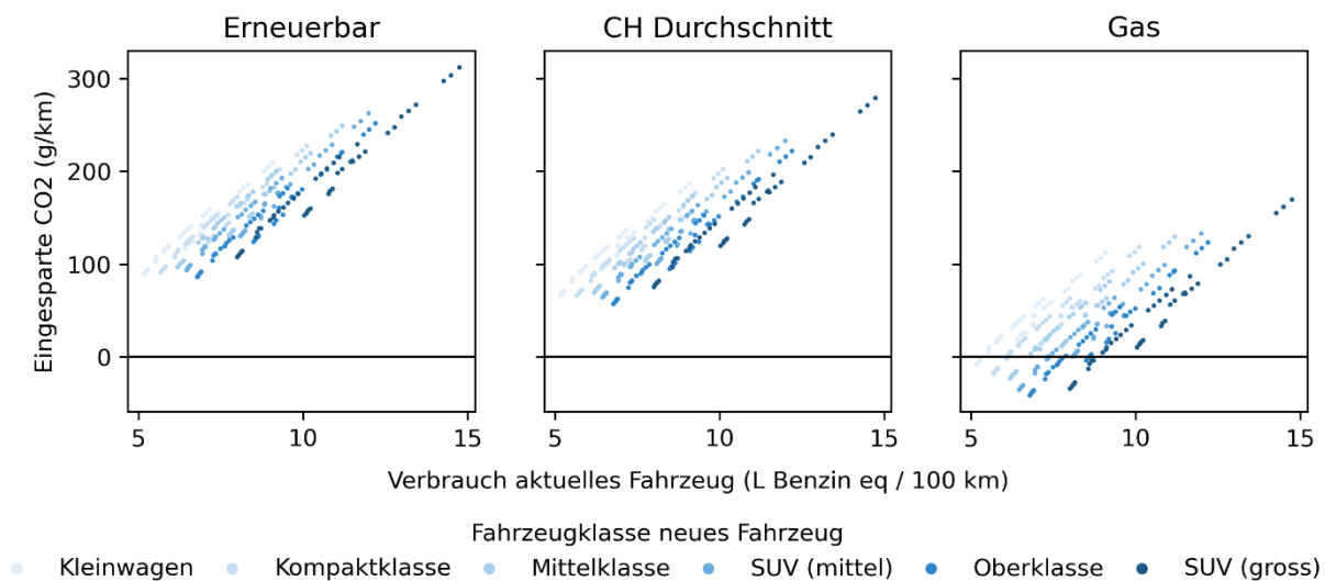
Abbildung 11: Sensitivität: Strommix. Datengrundlage: generische Fahrzeuge. Aktuelles Fahrzeug mit Verbrennungsmotor, Baujahr zwischen Jahr 2000 und 2022. Neues Fahrzeug elektrisch. Neues Fahrzeug in der gleichen Fahrzeugklasse wie das aktuelle Fahrzeug. Fahrleistung beim Entscheid 125'000 km. Lebensfahrleistung 200'000 km. Graphik INFRAS.
