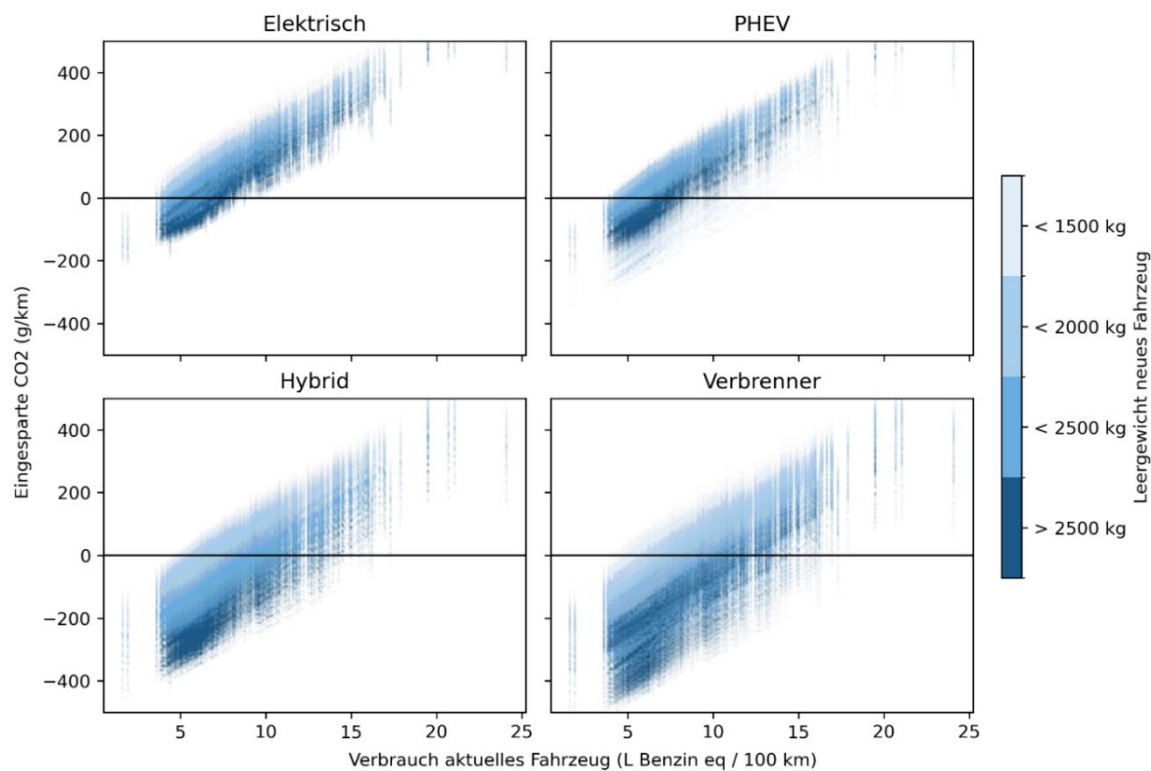
Abbildung 28: Eingesparte Treibstoffemissionen pro Kilometer für alle möglichen Fahrzeugkombinationen aus dem Verbrauchskatalog. Aktuelles Fahrzeug nur Verbrenner oder Hybrid. Neues Fahrzeug nur Modelle 2024. Antriebsart des neuen Fahrzeugs nach Quadrant. Schweizer Durchschnittstrommix. Lebensfahrleistung 200'000 km. Graphik INFRAS.
