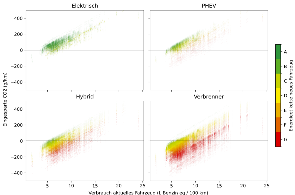
Abbildung 8: Eingesparte Treibstoffemissionen pro Kilometer für Fahrzeugkombinationen in der gleichen Fahrzeugklasse aus dem Verbrauchskatalog. Aktuelles Fahrzeug nur Verbrenner oder Hybrid. Neues Fahrzeug nur Modelle 2024. Antriebsart des neuen Fahrzeugs nach Quadrant. Schweizer Durchschnittsstrommix. Lebensfahrleistung 200'000 km. Graphik INFRAS.
