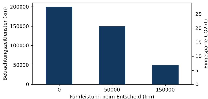
Abbildung 9: Sensitivität: Fahrleistung aktuelles Fahrzeug zum Zeitpunkt der Entscheidung. Vergleich: generisches Mittelklasse Benzinfahrzeug (Baujahr 2013) ersetzt durch generisches Mittelklasse Elektrofahrzeug (Baujahr 2023). Lebensfahrleistung 200'000 km. Graphik INFRAS.
