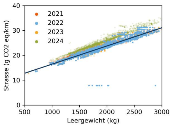
Abbildung 20: Regressionsanalyse der Strassenherstellungs- und Strassenwartungsemissionen. Daten aus dem Verbrauchskatalog. Regressionsbasis: Herstellungsjahr 2022. Graphik INFRAS.
