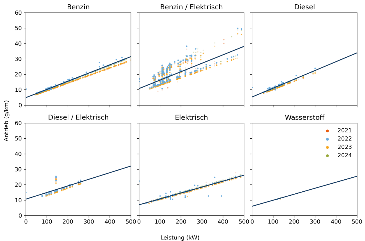
Abbildung 23: Regressionsanalyse der Antriebsherstellungsemissionen. Daten aus dem Verbrauchskatalog. Regressionsbasis: Herstellungsjahr 2022. Graphik INFRAS.
