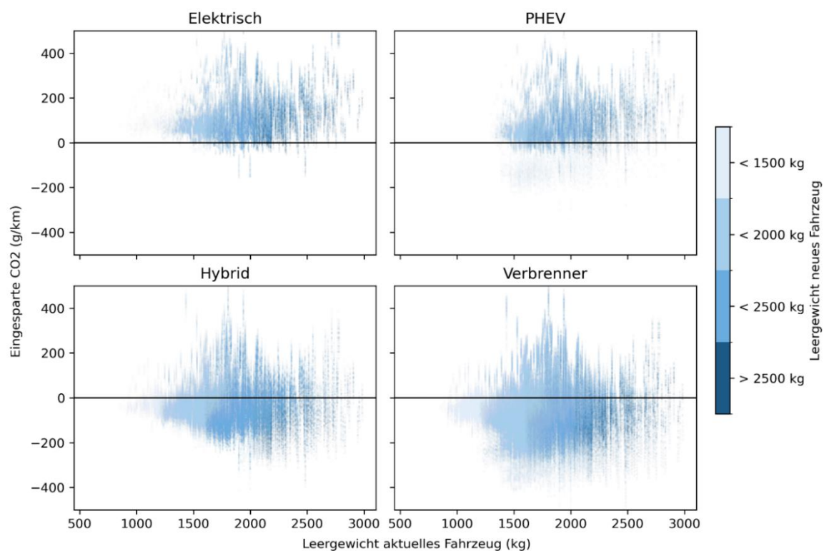
Abbildung 29: Eingesparte Treibstoffemissionen pro Kilometer für Fahrzeugkombinationen aus dem Verbrauchskatalog mit ähnlichem Leergewicht (+/- 20% Leergewicht). Aktuelles Fahrzeug nur Verbrenner oder Hybrid. Neues Fahrzeug nur Modelle 2024. Antriebsart des neuen Fahrzeugs nach Quadrant. Schweizer Durchschnittstrommix. Lebensfahrlleistung 200'000 km. Graphik INFRAS.
