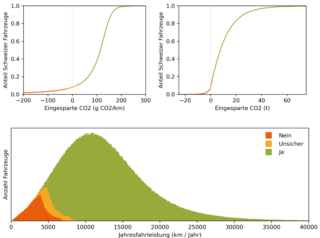
Abbildung 13: Hochrechnungsergebnisse. Verteilung der Fahrzeuge der Schweizer Flotte und die möglichen Treibhausgaseinsparungen, die ein Ersatz durch ein Elektroauto derselben Fahrzeugklassen mit sich bringen würde. Fahrzeugdaten: IVZ, LCA-Daten: generische Fahrzeuge. Graphik INFRAS
