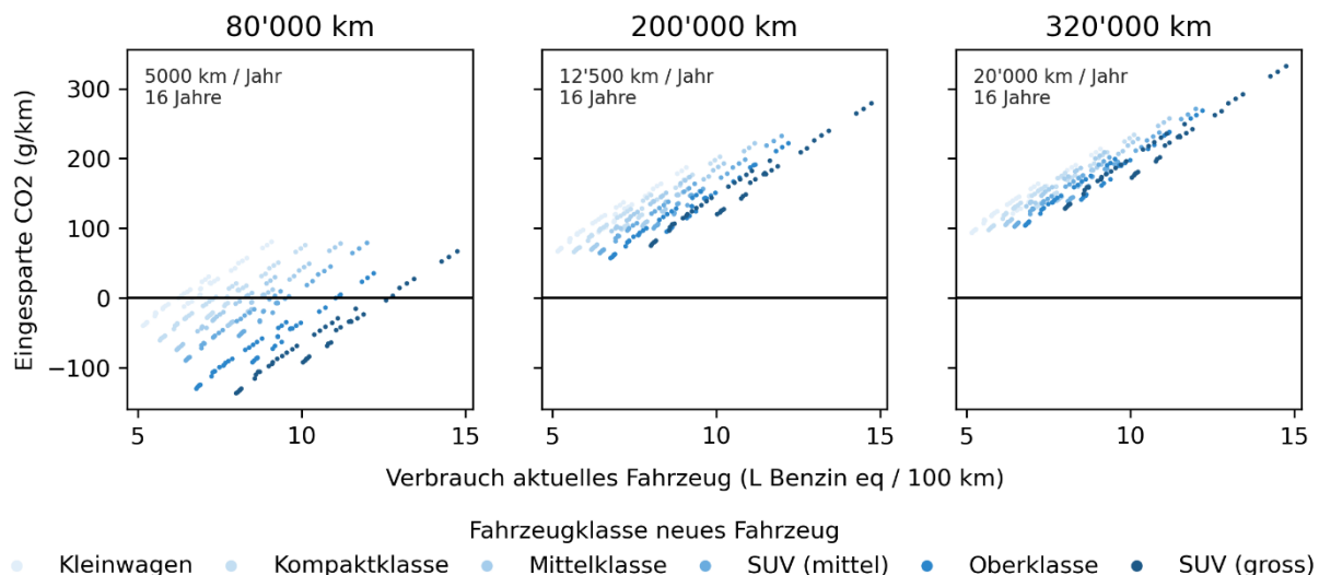
Abbildung 10: Sensitivität: Lebensfahrleistung neues Fahrzeug. Datengrundlage: generische Fahrzeuge. Aktuelles Fahrzeug mit Verbrennungsmotor, Baujahr zwischen 2000 und 2022. Neues Fahrzeug elektrisch, mit Schweizer Durchschnittstrommix geladen. Neues Fahrzeug in der gleichen Fahrzeugklasse wie das aktuelle Fahrzeug. Fahrleistung beim Entscheid 125'000 km. Graphik INFRAS.
