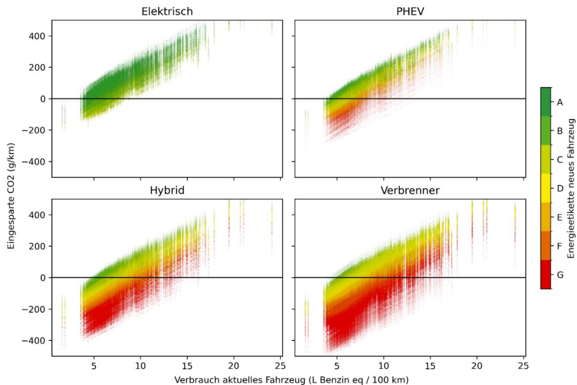
Abbildung 26: Eingesparte Treibstoffemissionen pro Kilometer für alle möglichen Fahrzeugkombinationen des Verbrauchskatalogs. Aktuelles Fahrzeug nur Verbrenner oder Hybrid. Neues Fahrzeug nur Modelle 2024. Antriebsart des neuen Fahrzeugs nach Quadrant. Schweizer Durchschnittsstrommix. Lebensfahrleistung 200'000 km. Graphik INFRAS. Wenn das neue Fahrzeug elektrisch angetrieben wird, aber die Fahrzeugklasse nicht unbedingt gleich sein muss, ergibt sich in rund 77% aller möglichen Fahrzeugkombinationen eine positive Treibhausgasbilanz. In den 23% der Fälle, in denen sich ein Umstieg nicht lohnt, ist das bisherige Fahrzeug fast immer klein und überdurchschnittlich effizient, während das neue Elektroauto ein grösseres Modell mit grosser Batterie und überdurchschnittlichem Verbrauch ist.
