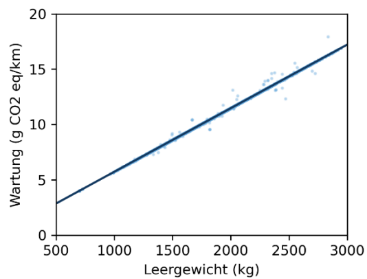
Abbildung 25: Regressionsanalyse der Wartungsemissionen. Daten aus dem Verbrauchskatalog. Regressionsbasis: Herstellungsjahr 2022. Graphik INFRAS.
